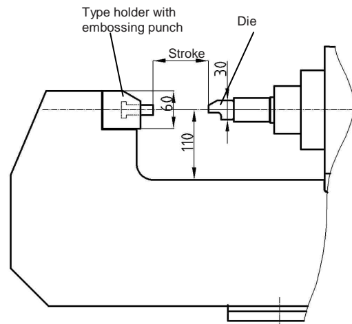
CBxx-Serie zum Prägen (mit Typenhalter)
